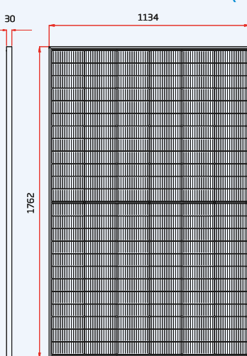
Frontansicht
